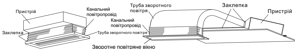
Режим установки нижнього забірника повітря
